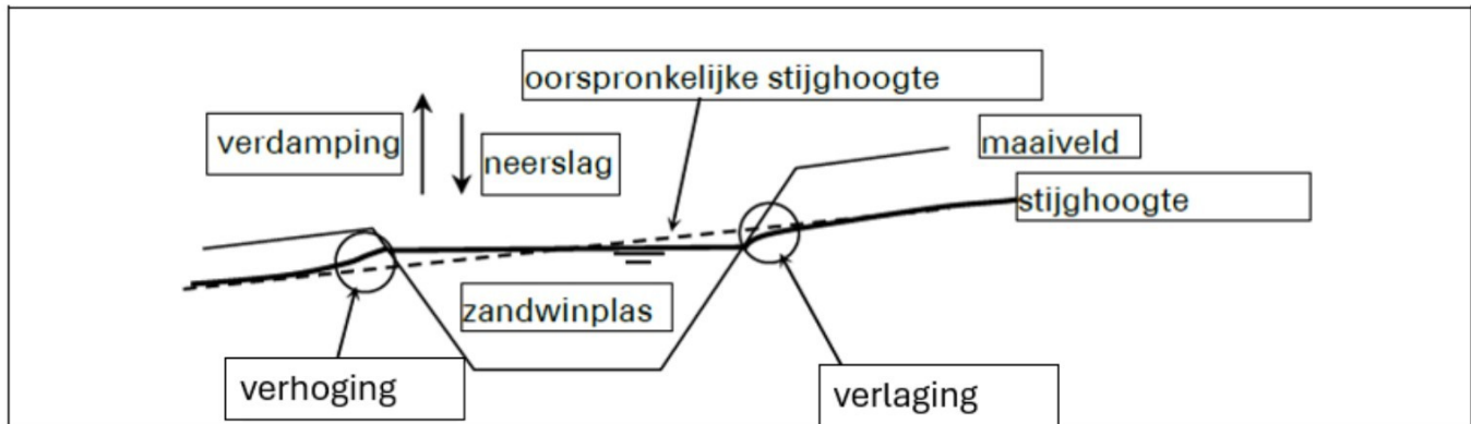
Figuur 3-2 Schematische weergave beïnvloeding stijghoogtestroming door zandwinplas (uit: Geohydrologische effectenstudie - Verdieping zandwinning Weperpolder te Oosterwolde (Wiertsema & Partners, 2023))
