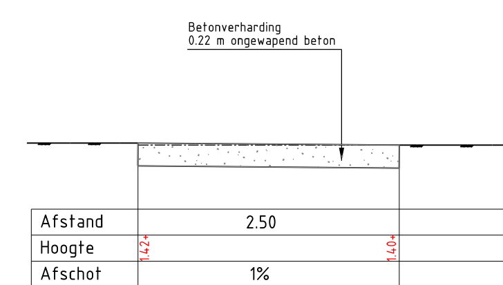
Doorsnede A-A Schaal 1:50
