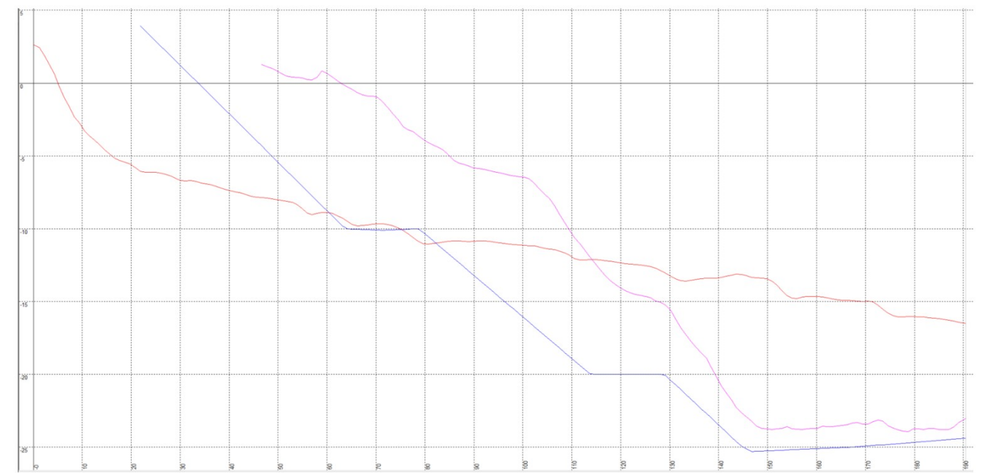
Lijn_6 (Mintgroen) (Rood = peiling bres 7-11-23, Roze = peiling 31-10-23, Blauw = ontwerp Inberg V4v2)
