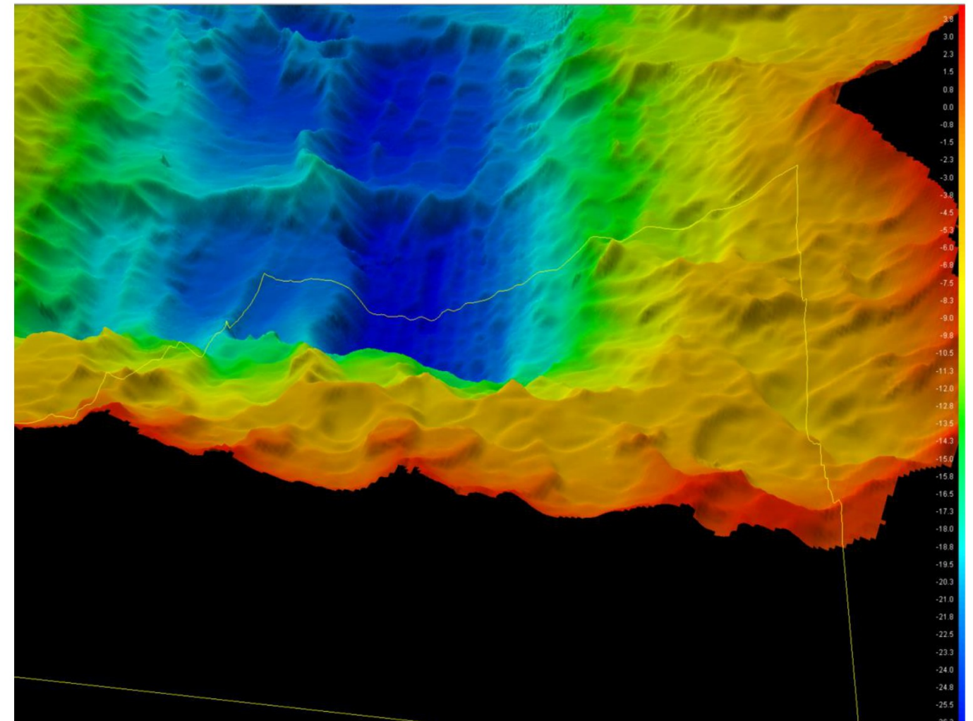
5.2 Peiling voor bresval, 31-10-23
