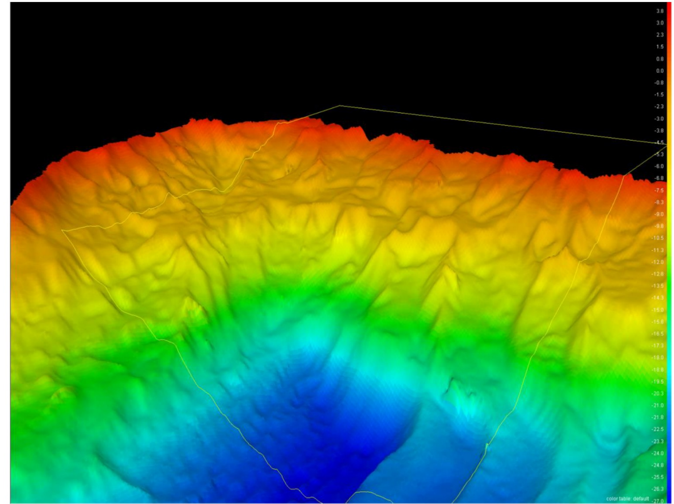
4.2 Peiling voor bresval, 31-10-23
