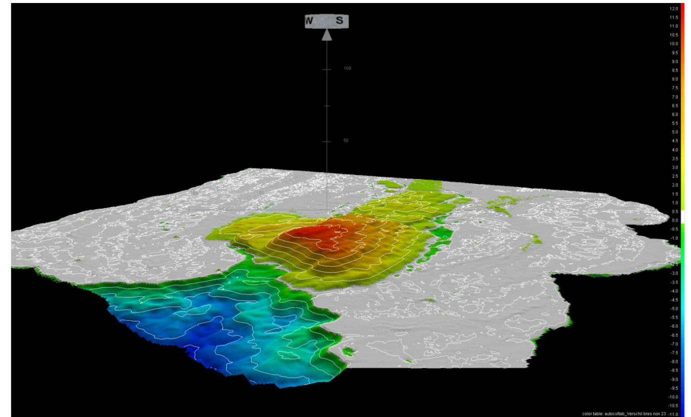
Figuur 6: Verschillenkaart peiling bres t.o.v. peiling 31-10-23 3D
