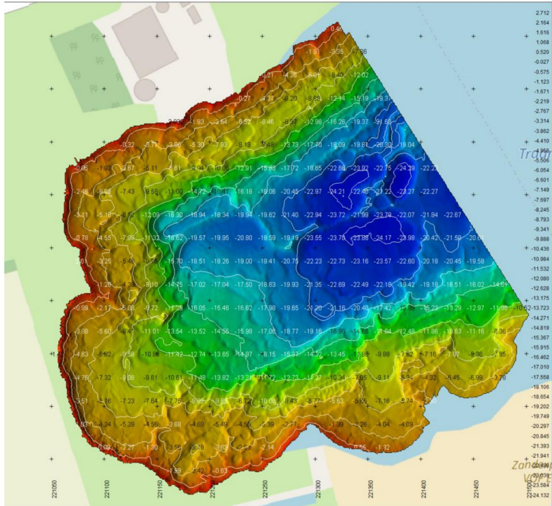
Figuur 1: Bres, peiling 7-11-23
