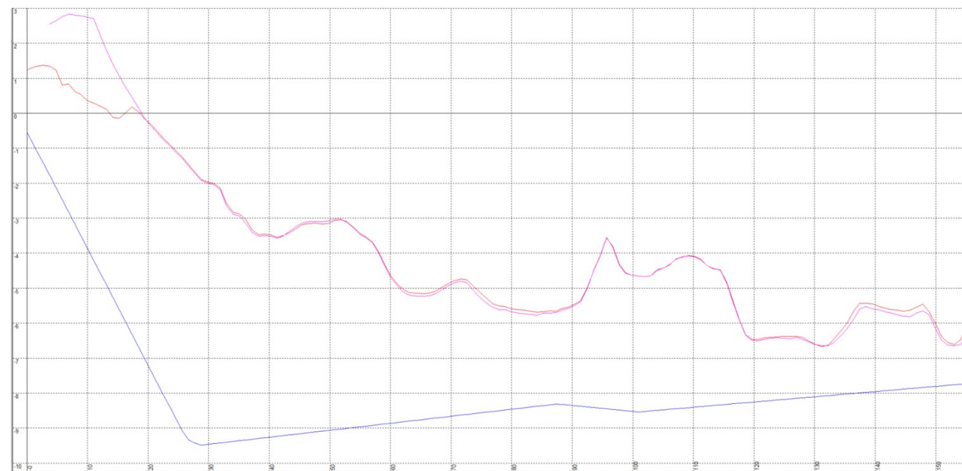
Lijn_12 (Donkerpaars) (Rood = peiling bres 7-11-23, Roze = peiling 31-10-23, Blauw = ontwerp Inberg V4v2)
