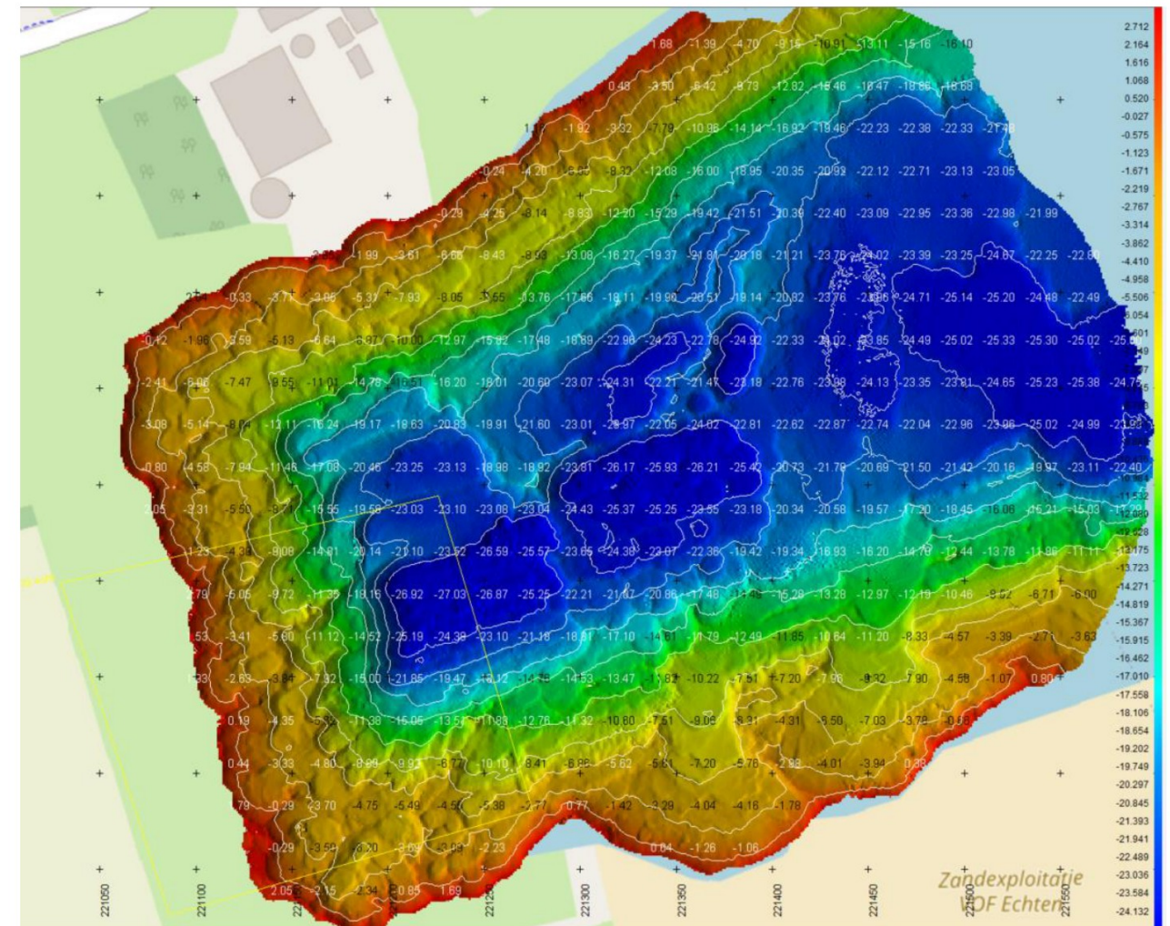
Figuur 2: Peiling 31-10-2023, voor bresval
