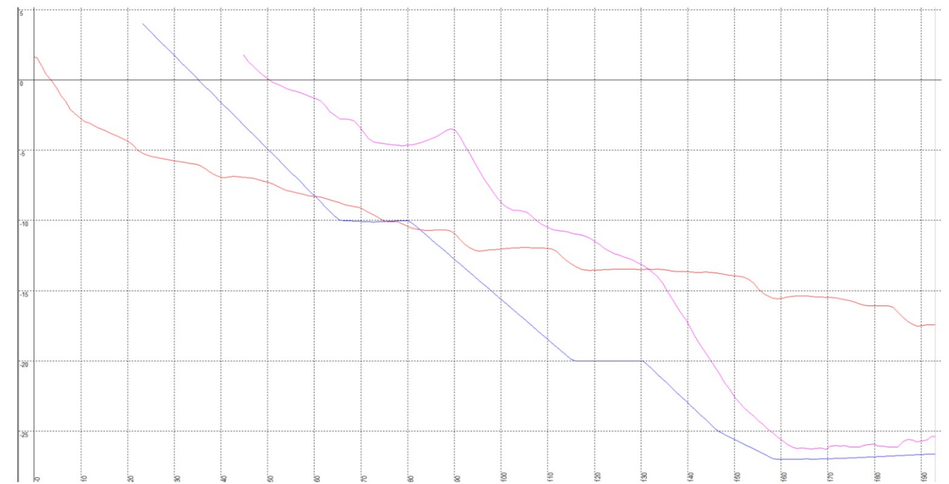
Lijn_6 (Mintgroen) (Rood = peiling bres 7-11-23, Roze = peiling 31-10-23, Blauw = ontwerp Inberg V4v2)
