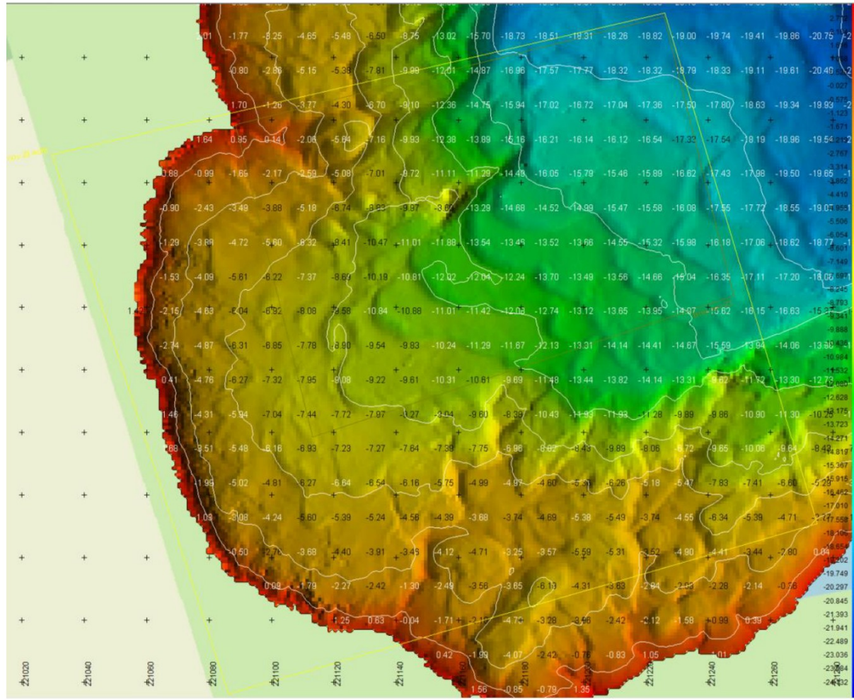
Figuur 3: Bres, peiling 7-11-23, ingezoomd
