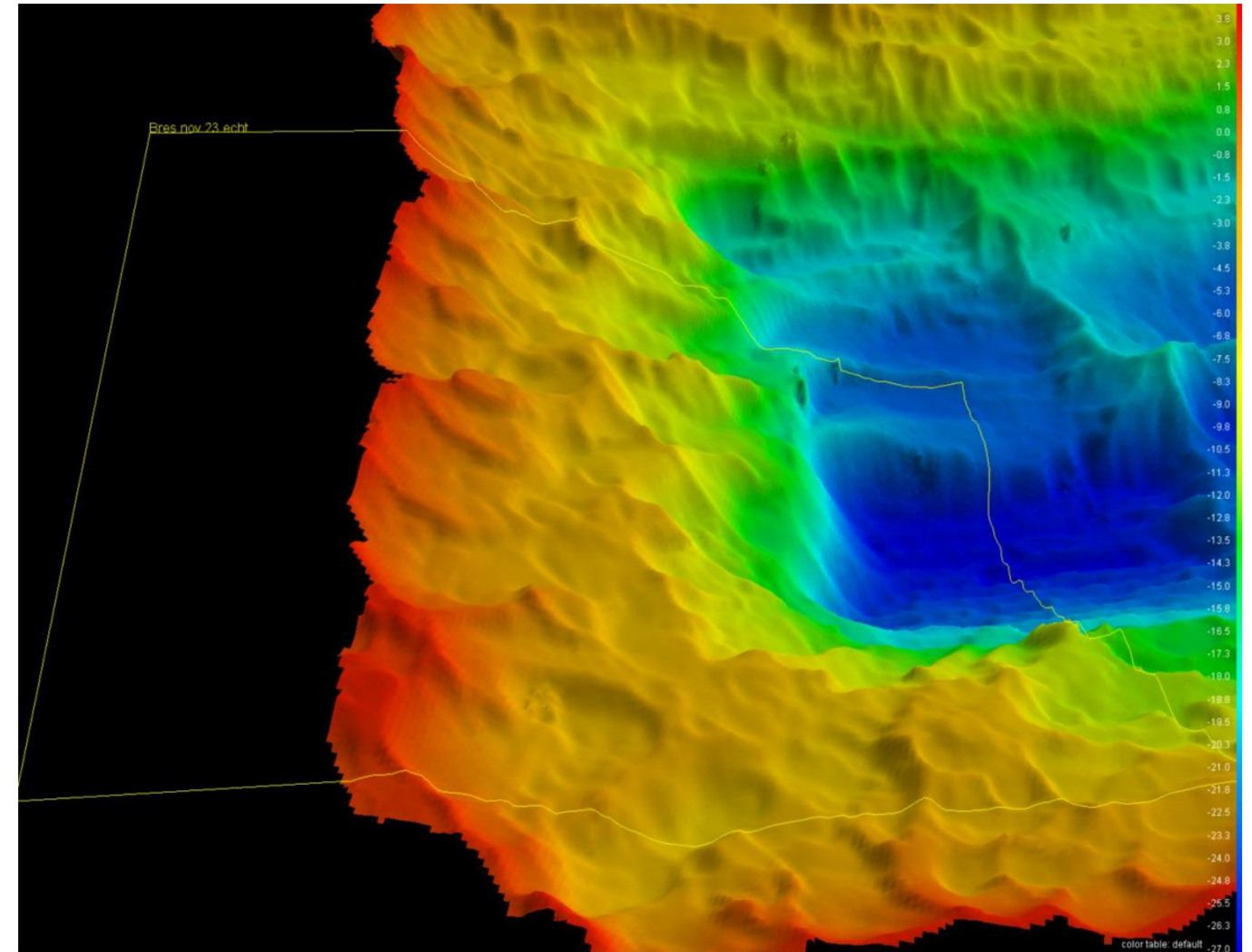
6.2 Peiling voor breval, 31-10-23
