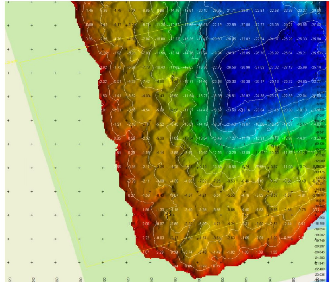
Figuur 4: Peiling 31-10-2023, ingezoomd
