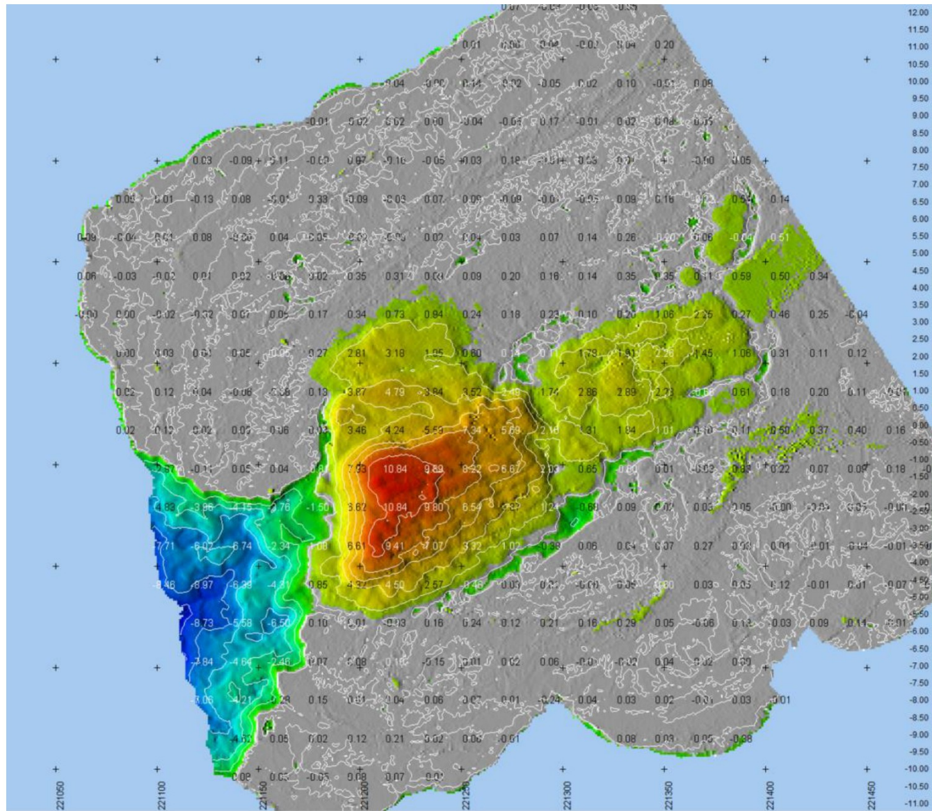
Figuur 5: Verschillenkaart peiling bres t.o.v. peiling 31-10-23
