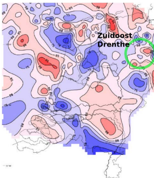
Figuur 3.4: temperaturen op 2000m
